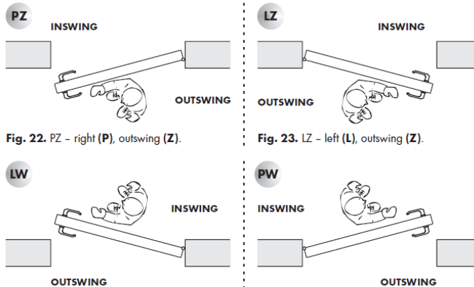
Verticale en horizontale doorsnede AW40-2 openslaande deur. Aluprof MB60 profiel systeem MET thermische onderbreking. Kan zowel buiten – als binnendraaiend geleverd worden.
