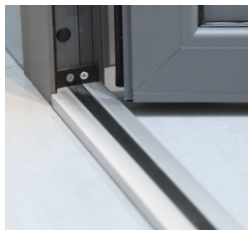
13 Aluminium dorpel met thermische onderbreking
