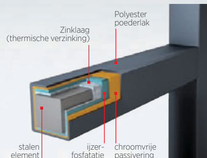
Doorsnede van een beveiligd element in het DUPLEX systeem
